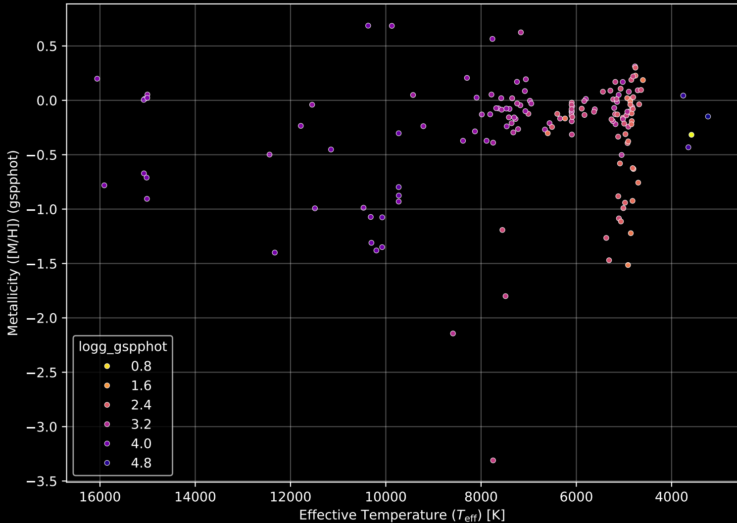
APOGEE DR17 Field: [113+04] Stellar Population Parameters (n= 156)
